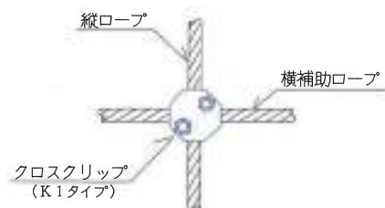
D部詳細図
