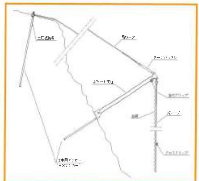
土中用支柱
