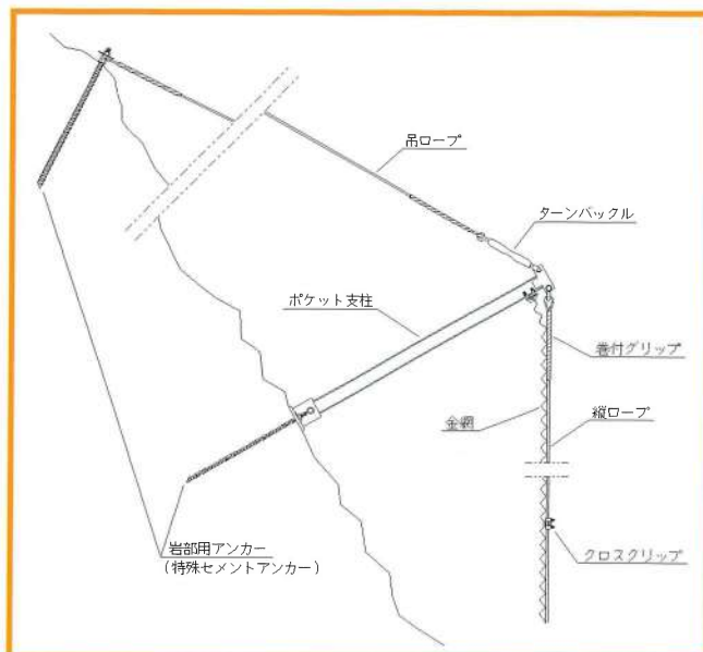
岩部用支柱
