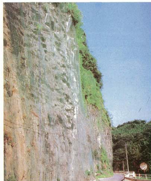
落石防護網(ロックネット)
