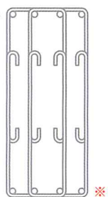
〔重ね継手〕
