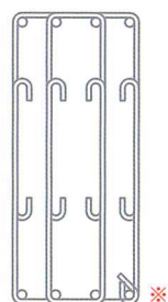
〔重ね継手+L形状〕
