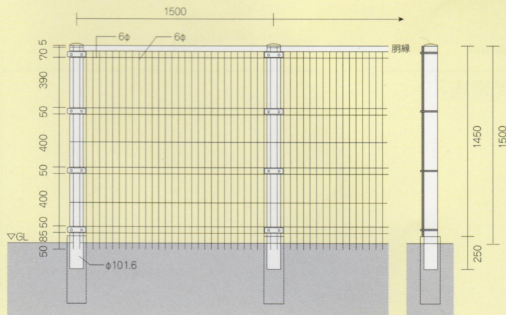
積雪地用フェンスGE2-4002
